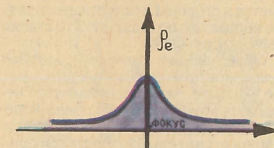
Рис. 1. Уменьшение плотности электронного газа ( n_e ) от центра к периферии лазерной мишени.
