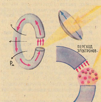
Рис. 4. Механизм возбуждения лазерной ЭДС в зазоре кольца.
