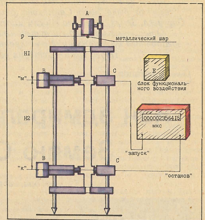
Схема прибора для измерения скорости падения тел.
