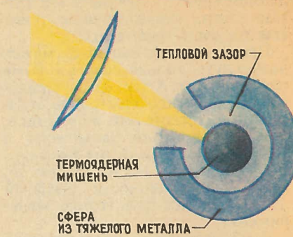
Рис. 6. Лазерная мишень в тяжелой металлической оболочке для использования эффекта самосжатия плазмы за счет спонтанных магнитных полей.
