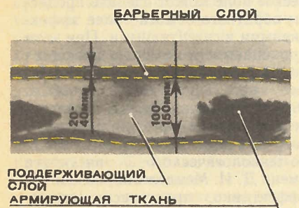
Схема и микрофотография дублированной фторопластовой мембраны.
