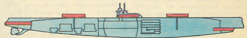
схемы эскизных проектов к конкурсу 11 июля 1909 г.
