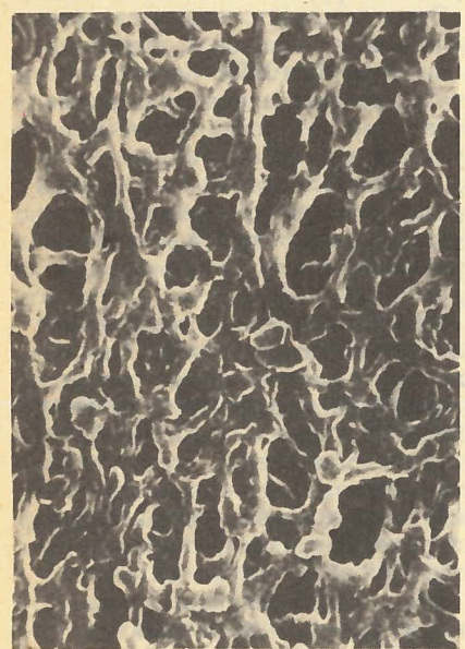
Микрофильтрующая ацетатная мембрана в электронном микроскопе.
