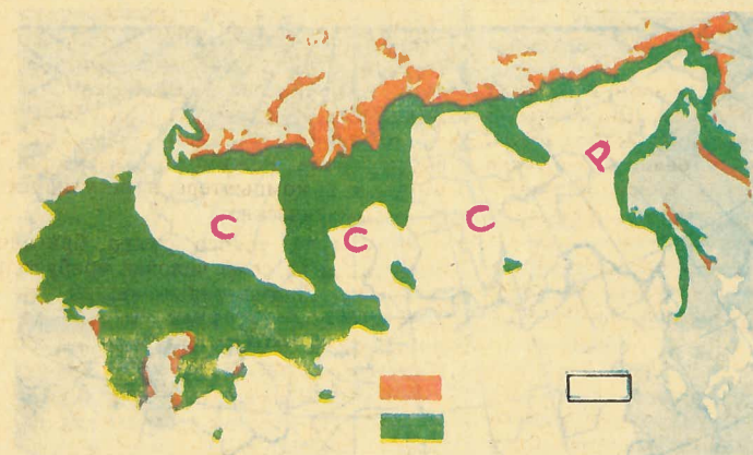
На этой карте выделены зоны с различными среднегодовыми скоростями ветра на высоте 10 м от земли: свыше 6 м/с (оранжевый цвет), 4—6 м/с (зеленый цвет), менее 4 м/с (белая зона).
