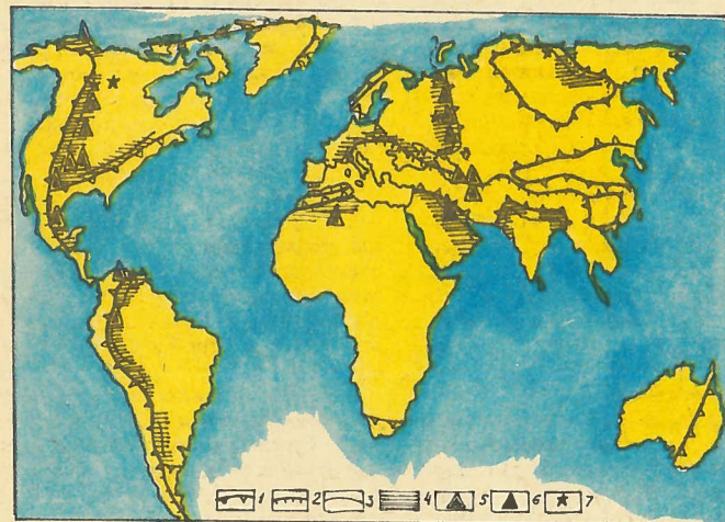
Нефтегазоносность передовых прогибов Земли
