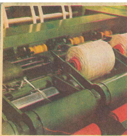
5. Узел автоматики ровничной машины. Схема работы узла (внизу): 1. Бобина заполнена. 2. Съем бобины. 3. Захват пустой катушки. 4. Установка пустой катушки.
