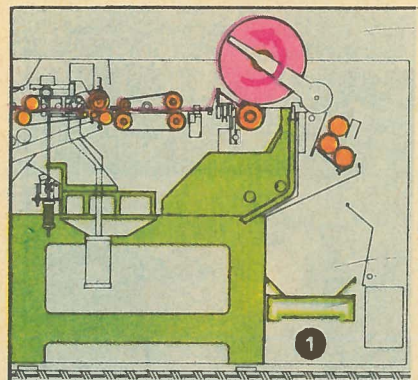
5. Узел автоматики ровничной машины. Схема работы узла (внизу): 1. Бобина заполнена. 2. Съем бобины. 3. Захват пустой катушки. 4. Установка пустой катушки.
