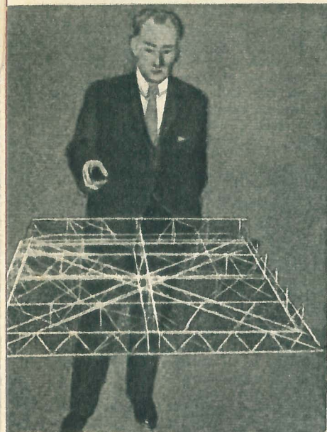
Майор ВВС США де Северский демонстрирует летающую модель ионокraftа.
