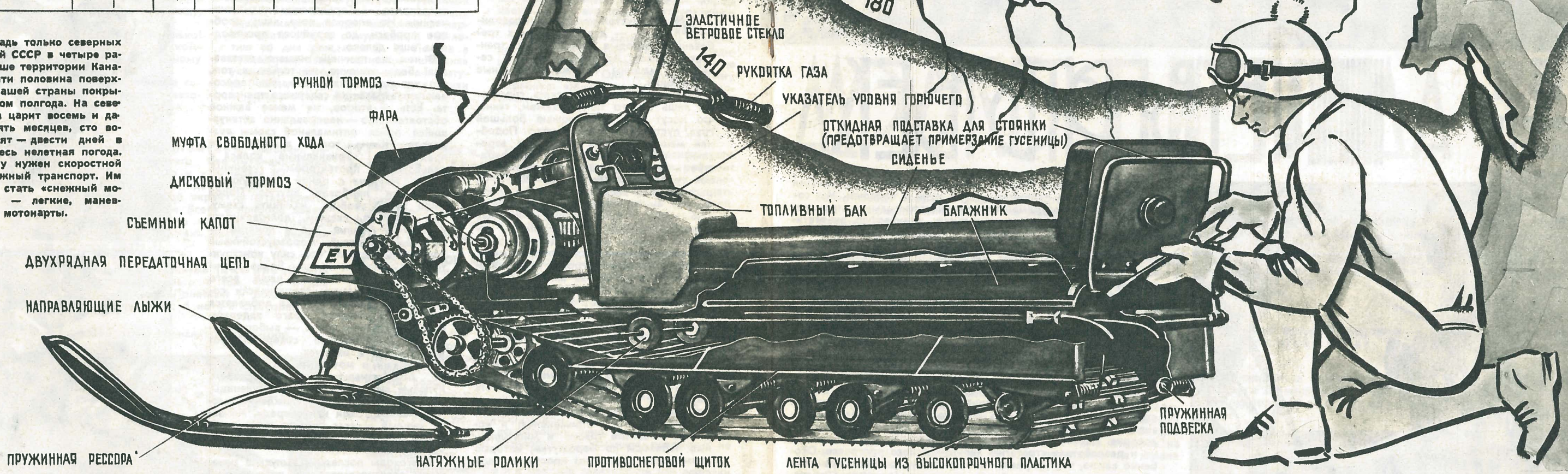
СНЕГОХОД „ЭВИНРУД“ (в разрезе)
