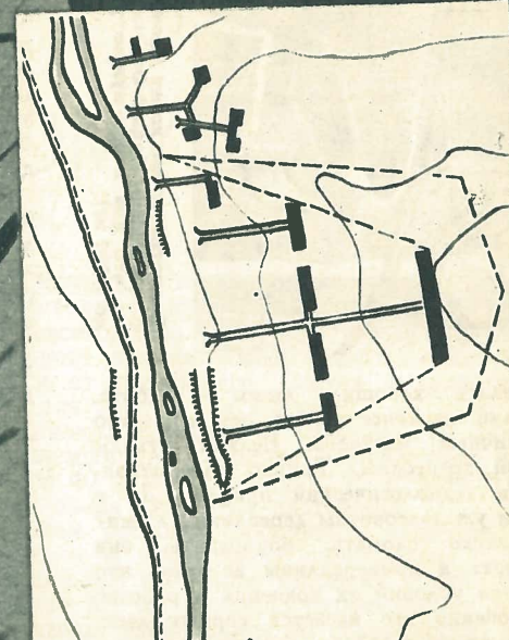
АЛМА-АТИНСКАЯ СЕЛЕЗАЩИТНАЯ ПЛОТИНА В РАЙОНЕ МЕДЕО СХЕМА РАСПОЛОЖЕНИЯ ЗАРЯДОВ
