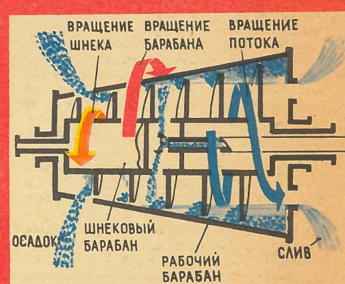
Шнековая осадительная центрифуга.
