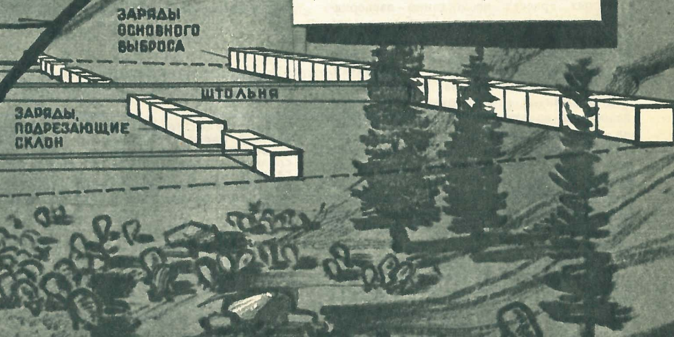
АЛМА-АТИНСКАЯ СЕЛЕЗАЩИТНАЯ ПЛОТИНА В РАЙОНЕ МЕДЕО СХЕМА РАСПОЛОЖЕНИЯ ЗАРЯДОВ
