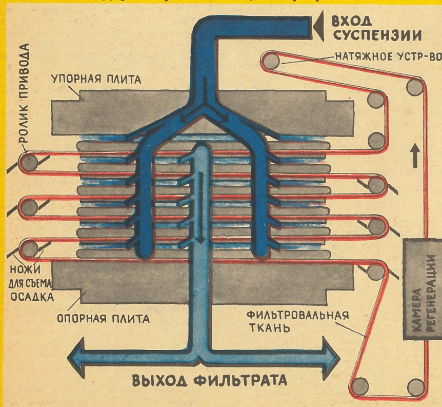
ФПАКМ — автоматический камерный модернизированный фильтр-пресс.
