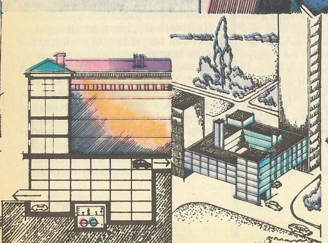
Общий вид одной из модификаций гаража ПУСЛАТ. Цифрами обозначены: 1 — вертикальные секции гаража, 2 — помещение с управляющей ЭВМ, 3 — комната отдыха, 4 — переход, 5 — въезды для легковых автомобилей, 6 — автостоянка, 7 — въезды для грузовых автомашин, 8 — монтируемые секции.
