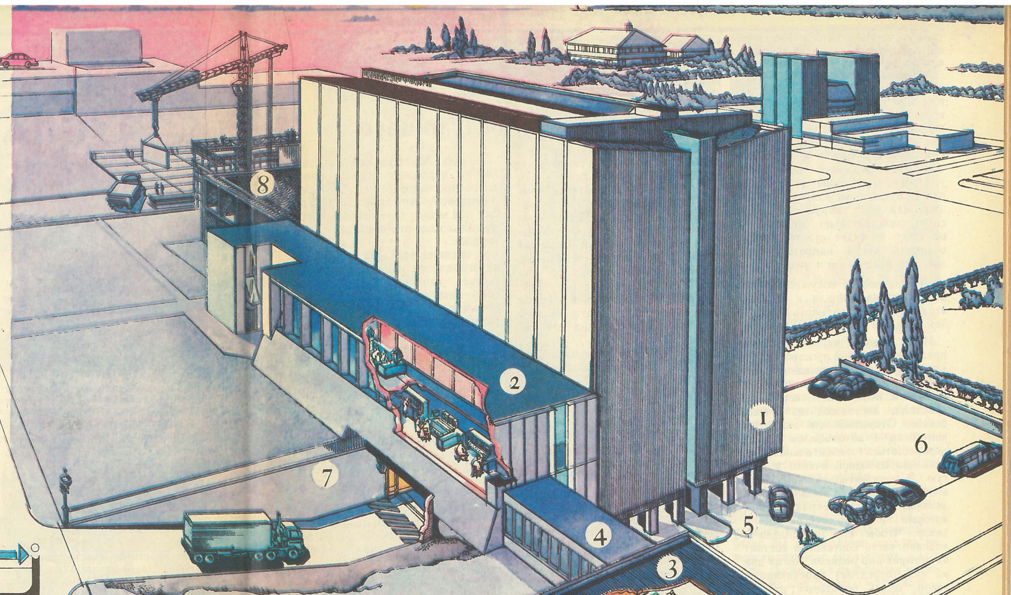
Общий вид одной из модификаций гаража ПУСЛАТ. Цифрами обозначены: 1 — вертикальные секции гаража, 2 — помещение с управляющей ЭВМ, 3 — комната отдыха, 4 — переход, 5 — въезды для легковых автомобилей, 6 — автостоянка, 7 — въезды для грузовых автомашин, 8 — монтируемые секции.
