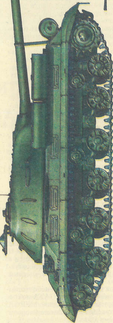
ИС-7. Опытный, изготовлен в 1948 г. Масса — 68 т, экипаж — 5 человек, длина — 7380 мм, ширина — 3400 мм, высота — 2480 мм. Вооружение — 130-мм пушка (боекомплект 28 снарядов), 12,7-мм спаренный с ней пулемет, шесть 7,62-мм пулеметов (четыре установлены вперед, на гусеничных полках и на бортах башни, управляют дистанционно), 12,7-мм зенитный пулемет на крыше башни (в походном положении складывался на ее левый борт). Бронирование — лоб башни — 210 мм, лоб корпуса — 150 мм. Мощность двигателя — 1050 л. с., скорость — 59 км/ч, запас хода — 300 км.
