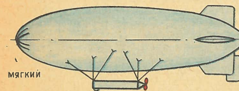
Варианты расположения силовой установки в нижней части фюзеляжа дирижабля.
