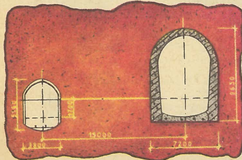
Схема тоннеля Байкальского.
