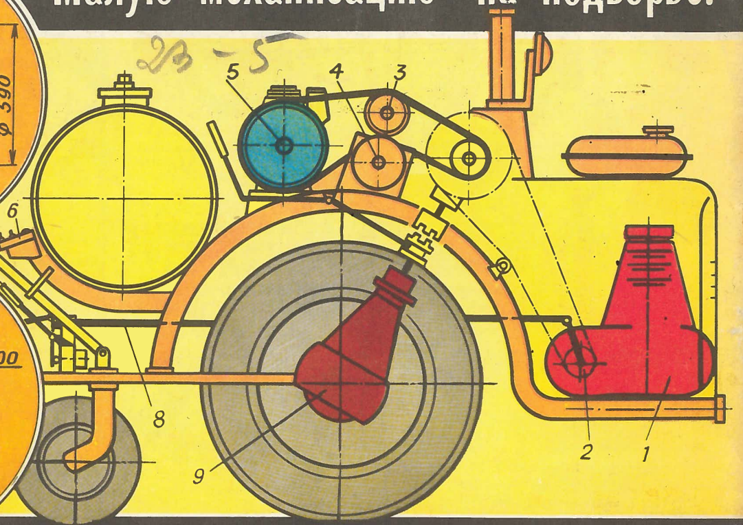
КИНЕМАТИЧЕСКАЯ СХЕМА ТРАКТОРА
