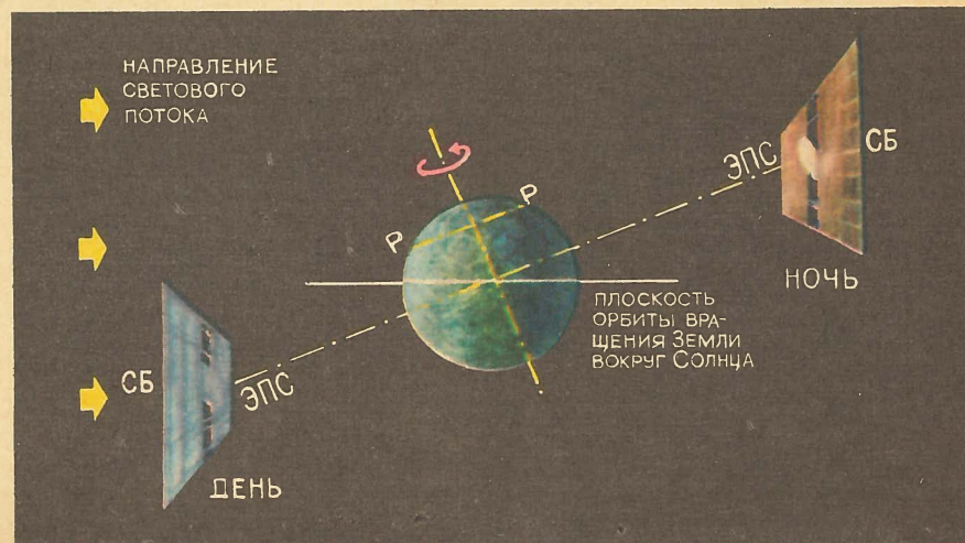
Дневное и ночное положение КЭС на околоземной орбите.
