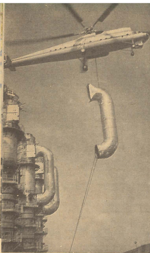
«Летающий» кран незаменим при реконструкции действующих цехов, когда традиционная грузоподъемная техника оказывается бессильной. Установку сирубберов и газоходов на Синарском трубном заводе выполняют специалисты треста «Востокметаллургмонтаж».
